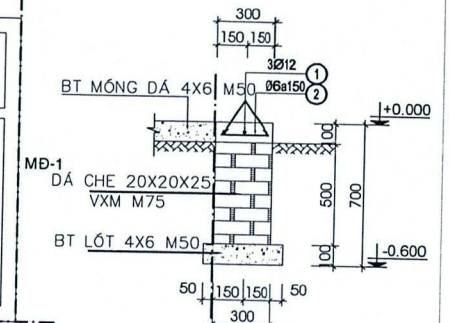
MÓNG MD1
