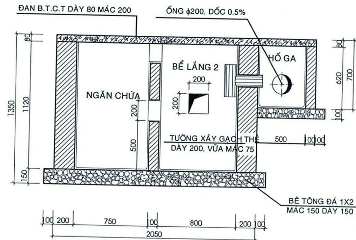
MẶT CẮT 1-1
