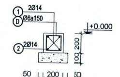
GM-2(200X200)
