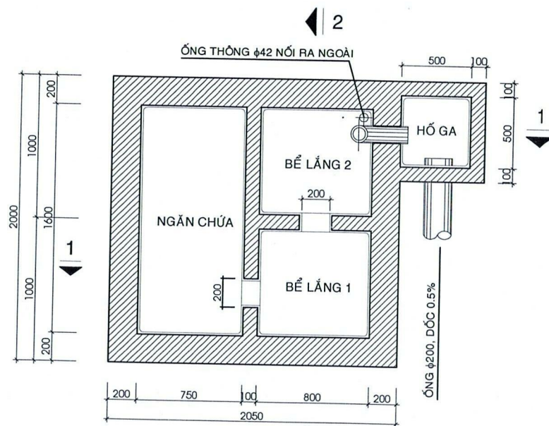
MẶT BẰNG HẠM TỰ HOẠI
