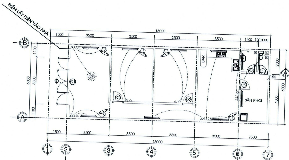
MẶT BẰNG ĐIỆN TẦNG TRỆT
