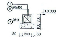
GM-1(200X200)
