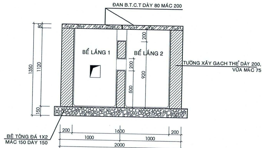
MẶT CẮT 2-2
