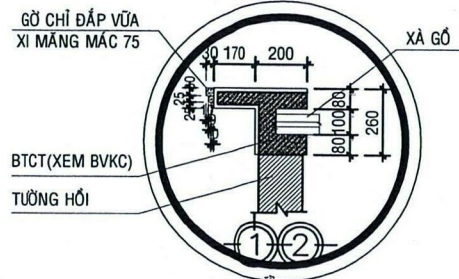
CHI TIẾT DIỀM MÁI TỶ LỆ : 1/5
