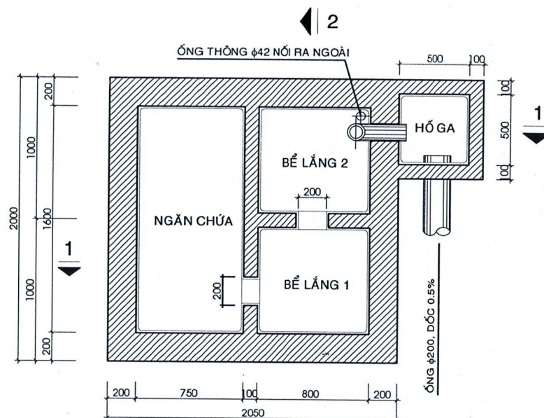
MẶT BẰNG HẦM TỰ HOẠI
