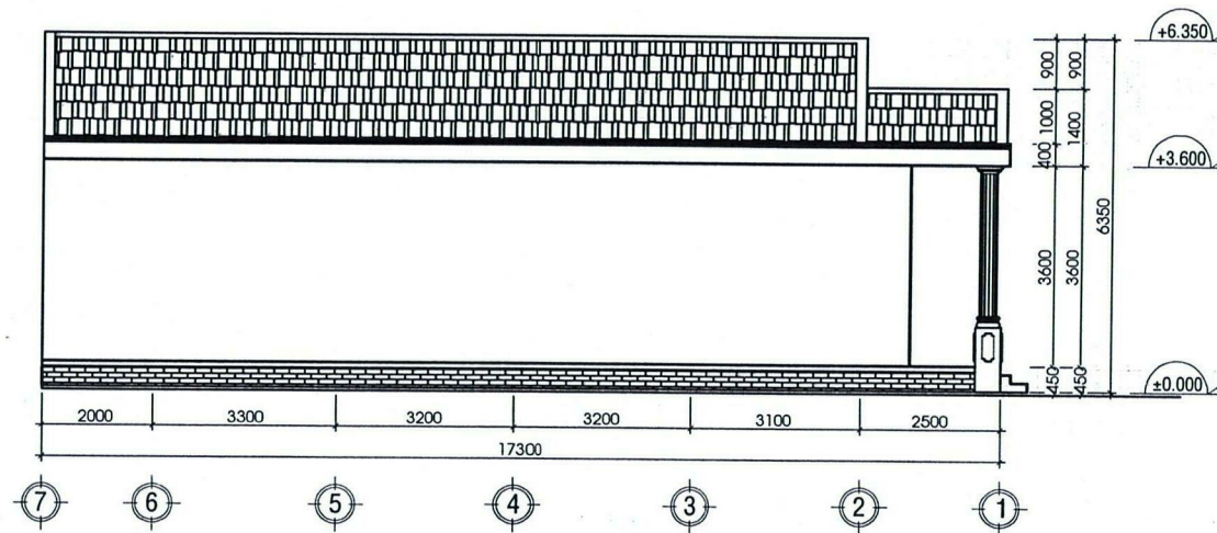
MẶT BÊN TRỰC 7-1 TỶ LỆ : 1/100
