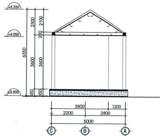
MẶT CẮT B-B TỶ LỆ : 1/100
