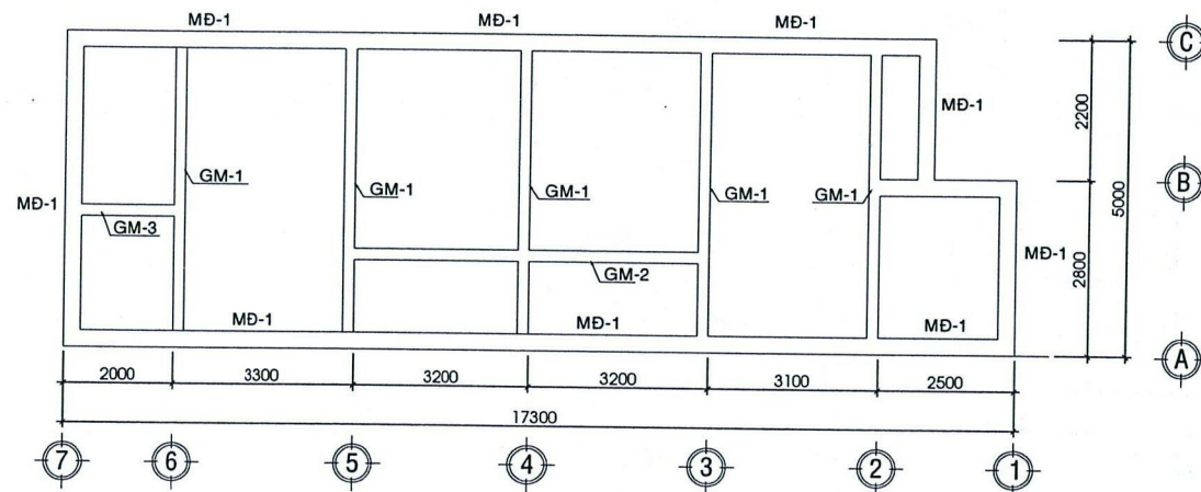
MẶT BẰNG MĐ, GM TL 1/100
