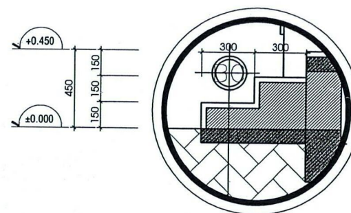
CHI TIẾT (CT01) TỶ LỆ : 1/20
