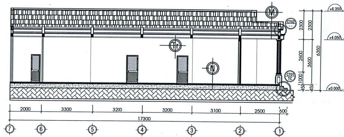
MẶT CẮT A-A TỶ LỆ : 1/100
