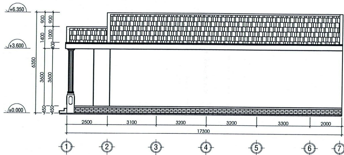
MẶT BÊN TRỤC 1-7 TỶ LỆ : 1/100
