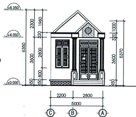
MẶT ĐƯƠNG CHÍNH TỶ LỆ : 1/100
