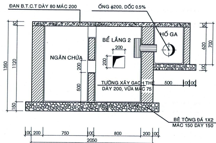
MẶT CẮT 1-1
