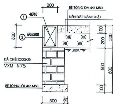
MÔNG MD1 TL.1/20.L=44M
