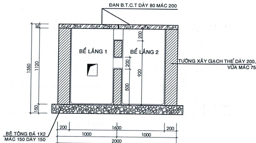
MẶT CẮT 2-2
